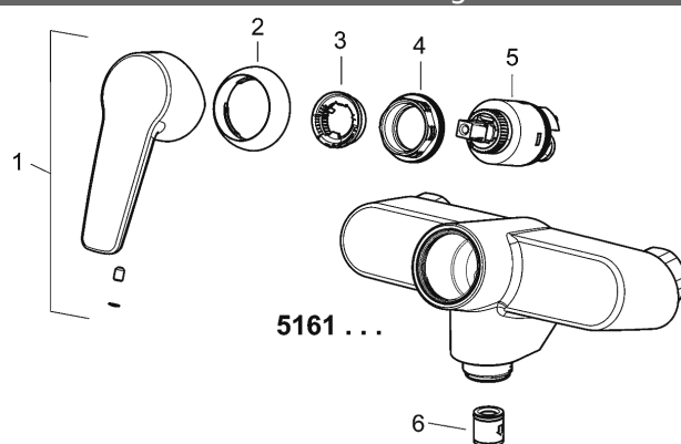
Producttekening
