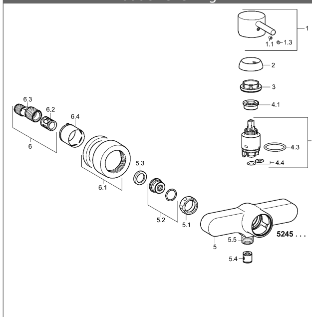
Producttekening
