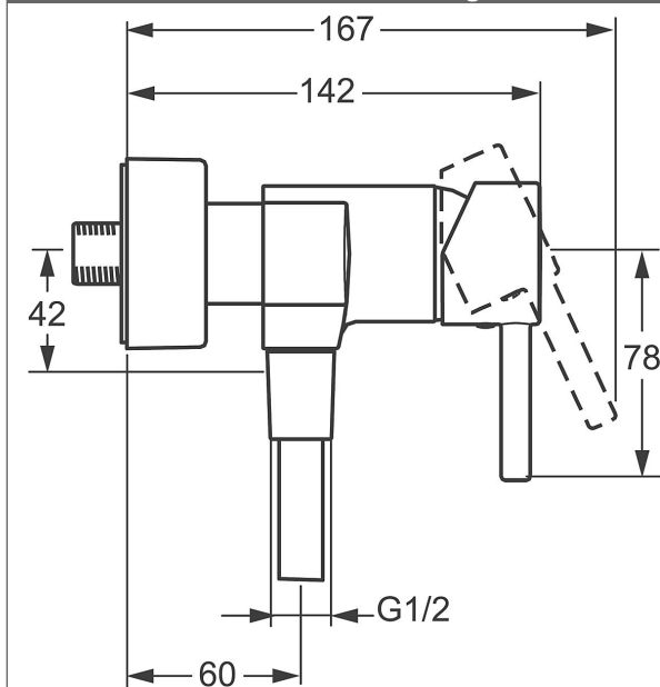
Producttekening
